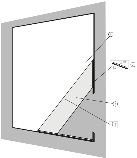
M597 Diagrama de instalación (M597) para Clipso SO Acoustic AB, aplicación en pared con perfiles PCC
