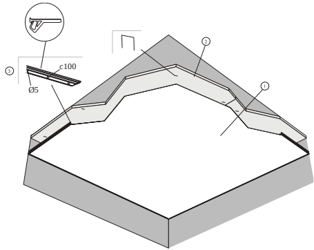
M596 Diagrama de instalación (M596) para Clipso SO Acoustic AB, aplicación en techos con perfiles PCW
