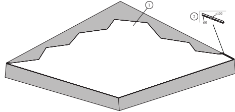
M598 Diagrama de instalación (M598) para Clipso SO Acoustic AB, aplicación en techos con perfiles PCC
